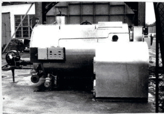
ASEA Sao Paulo Basilien. Helvatten panna Univer V-DE 40
